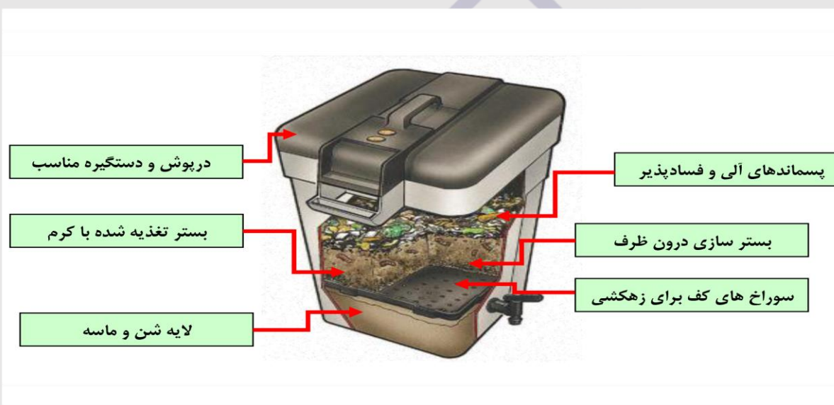
شکل (۸) - نمونه طرح شماتیک مخزن آماده سازی شده برای تهیه ورمی کمپوست
