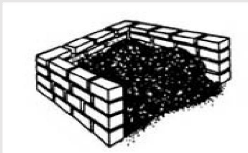
شکل (۴) - جایگاه ساخته شده از مصالح ساختمانی جهت تهیه بیوکمپوست خانگی
